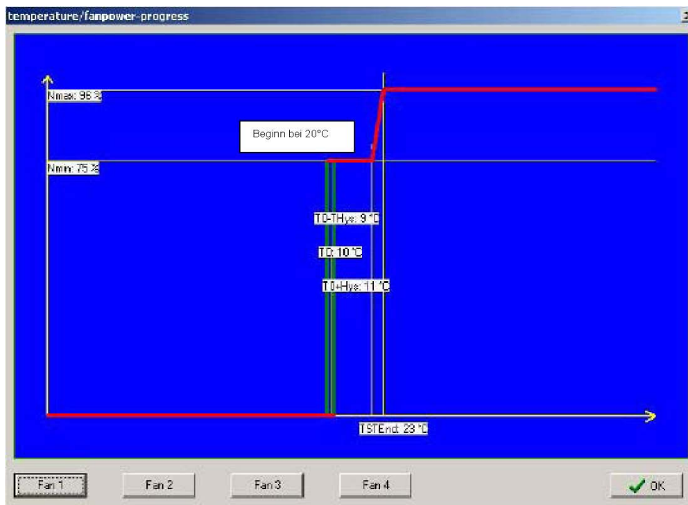
Kennlinie Lüfterregelung (Werkseinstellung)
